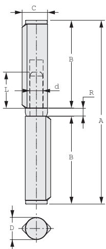
Výškově regulovatelný ocelový čep s kuličkovým ložiskem
