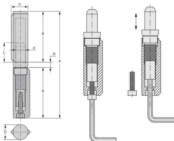
Výškově regulovatelný ocelový čep s kuličkovým ložiskem
