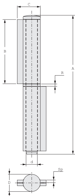
3 dílný – výsuvný čep s podložkou
