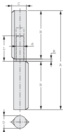
Mosazný čep a kuličkové ložisko
