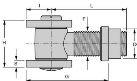
Pant k přivaření
