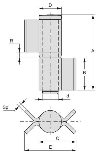
3 dílný, výsuvný čep - 2 mosazné podložky
