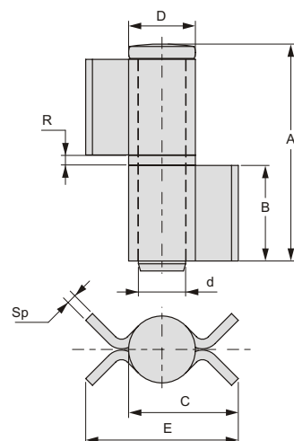
2 dílný, výsuvný čep - 1 mosazná podložka
