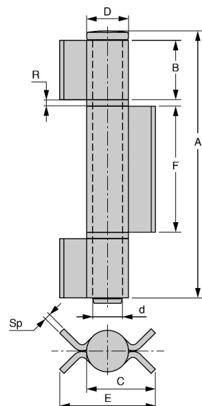
3 dílný, výsuvný čep - 2 mosazné podložky
